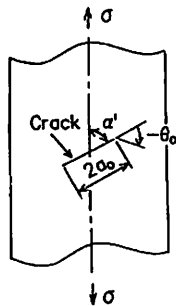
(a) 板平面で傾斜したき裂
