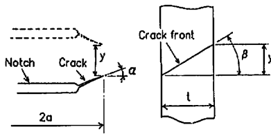
図 4 き裂傾斜角の定義
