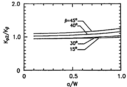
図11 応力拡大係数比 K_{p2}/K_{\beta} と無次元き裂長さ a/W の関係
