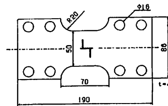
図 1 試験片形状と寸法 [mm]
