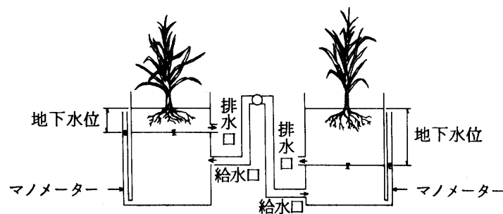
図-1 地下水位および給水方法
