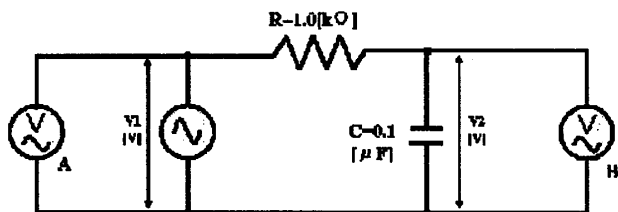
図1. 実験回路
