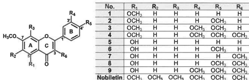
MRR に含有するメトキシフラボン (1-9)の構造
